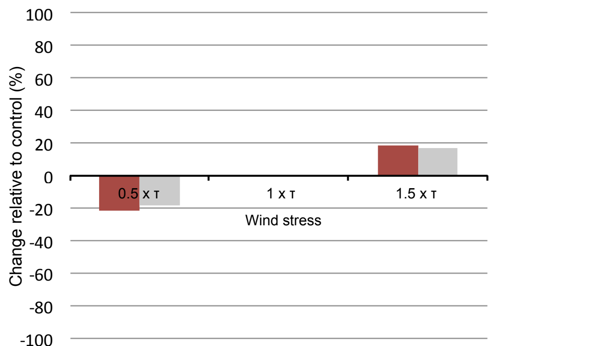
(d) Hypoxic volume
