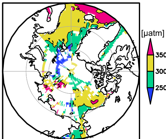
(d) p\text{CO}_{2w} (RMSD)
