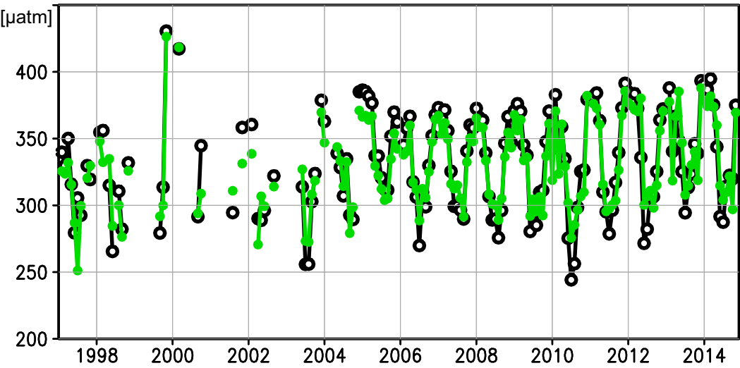
(b) p\text{CO}_{2w} (bias RMSD)
