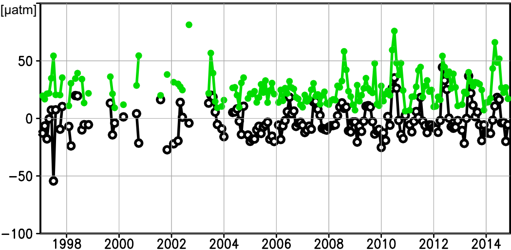
(b) p\text{CO}_{2w} (bias RMSD)
