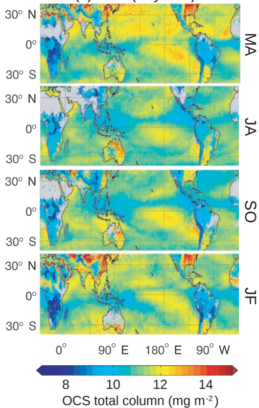
(c) IASI (daytime)
