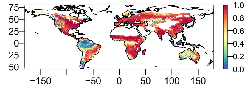
(d) R 2 between CSIF and SIF*
