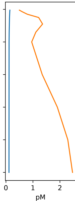
(c) Olig. Atl.
