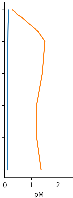
(b) Eq. Pac.
