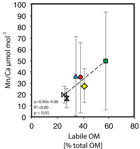
Melonis barleeanus
