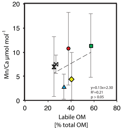
Uvigerina peregrina
