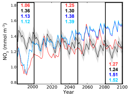
(d) Nitrate surface (0–200 m)
