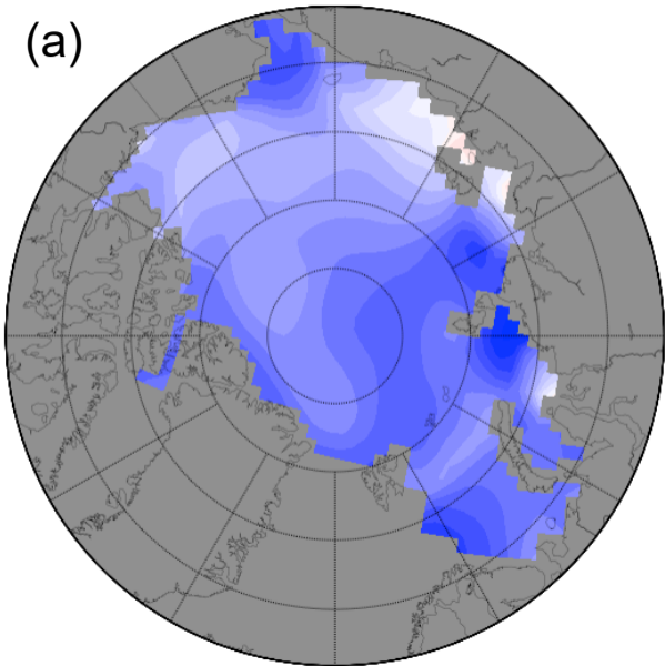
ORCA2
