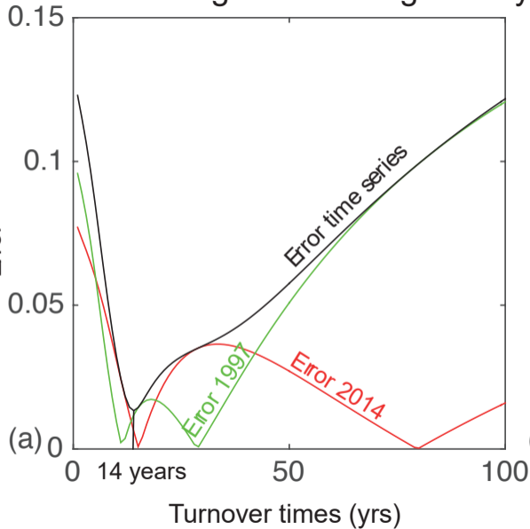
Beatenberg - Podzol organic layer
