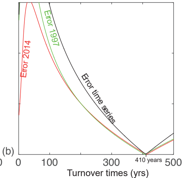
Beatenberg - Podzol 0–5 cm
