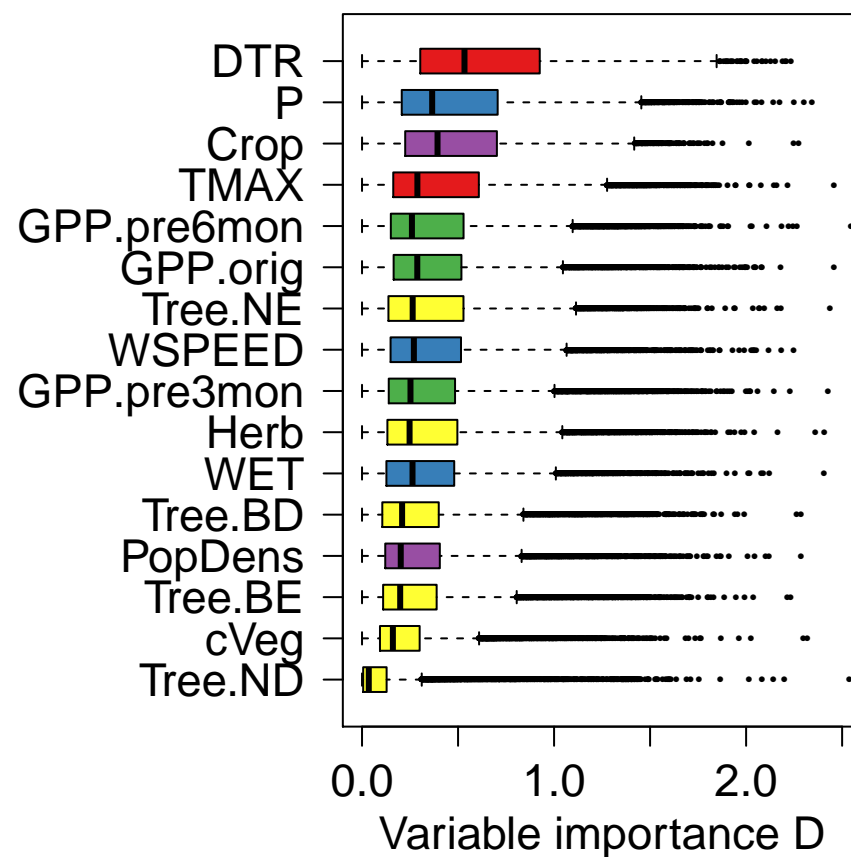
(d) Importance in RF.FireMIP
