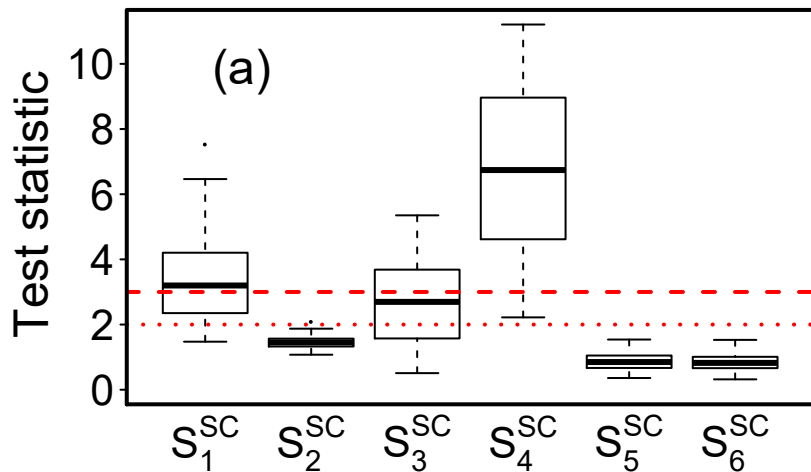
Haar variance
