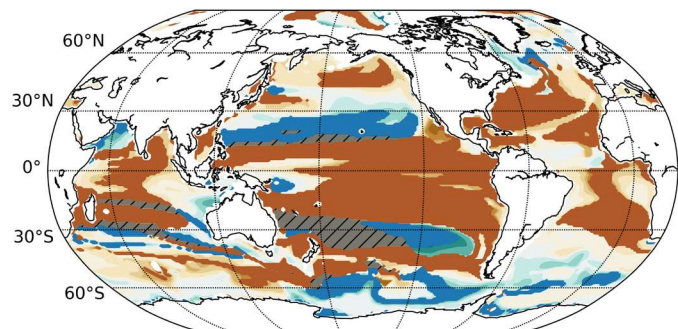
(d) IPSL-CM5B-LR
