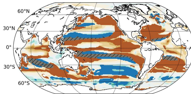
(h) MPI-ESM-LR
