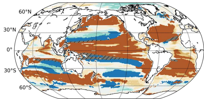
(g) MPI-ESM-MR
