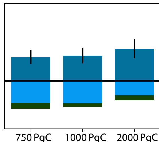
UVic ESCM 2.10
