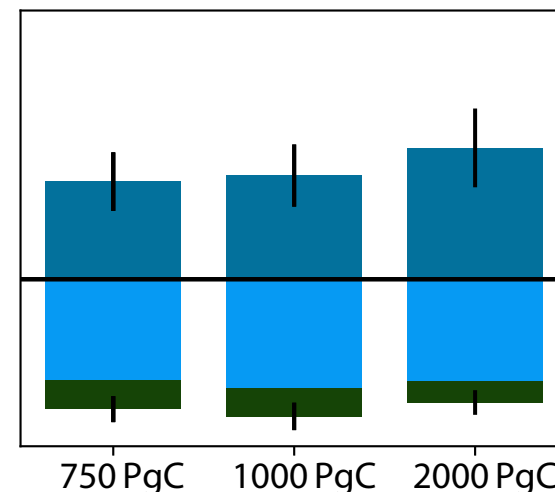
MESM
