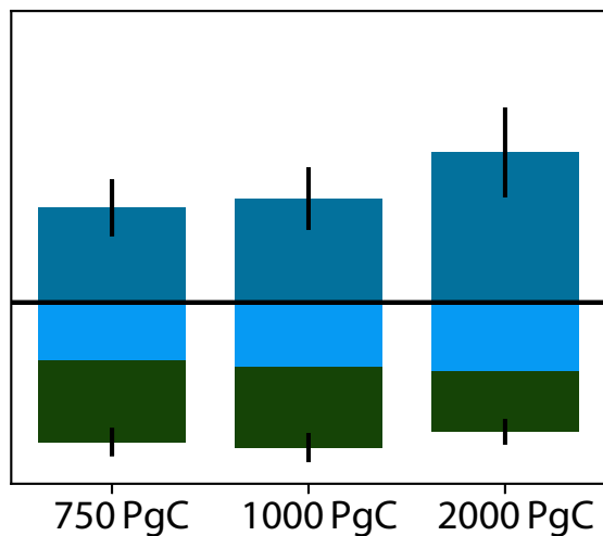
DCESS
