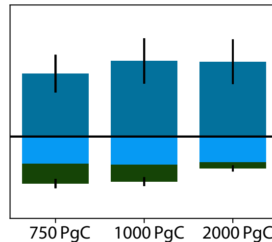
MESM
