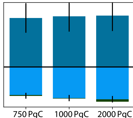
UVic ESCM 2.10
