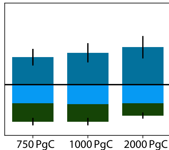
IAPRAS
