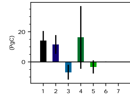
Cum. LASC (1750–2018)
