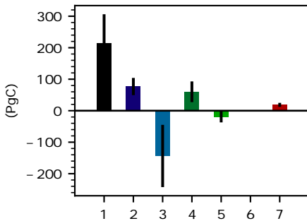
Cum. ELUC (1750–2018)
