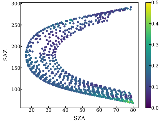
Fir NIRv
