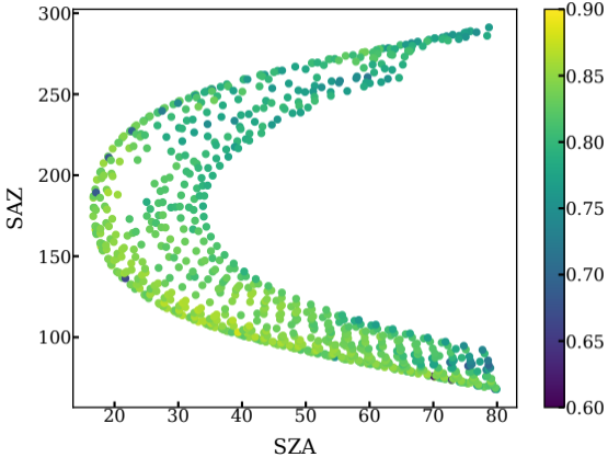
Fir NDVI
