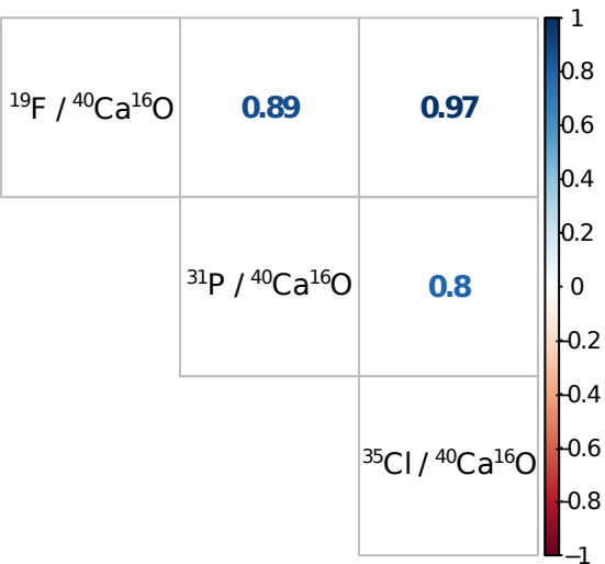
Ammonia tepida , n=40
