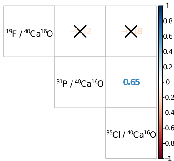
Sorites marginalis , n=45
