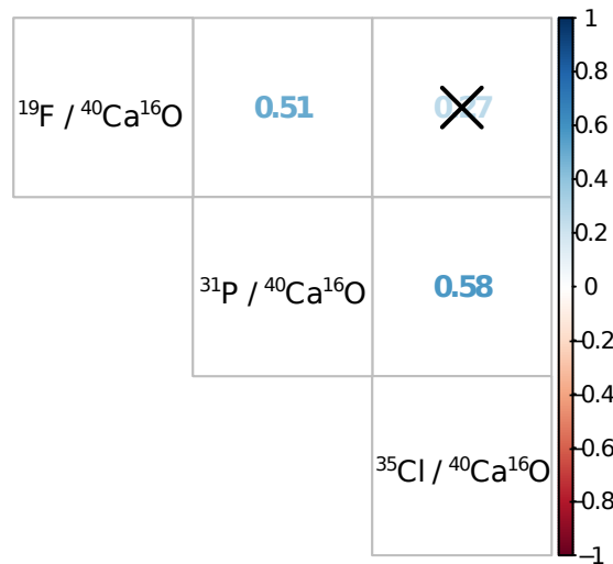
Amphistegina lessonii , n=47
