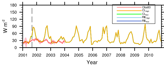
(d) Latent heat flux (logged)
