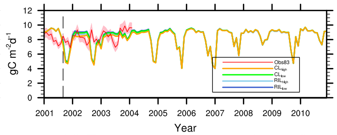
(d) Ecosystem respiration (logged)
