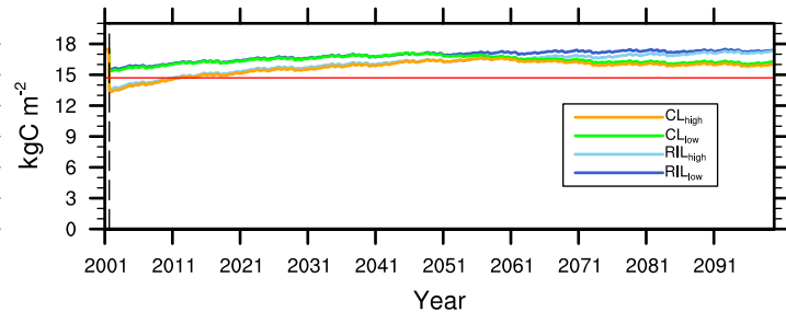
(d) Coarse woody debris (logged)
