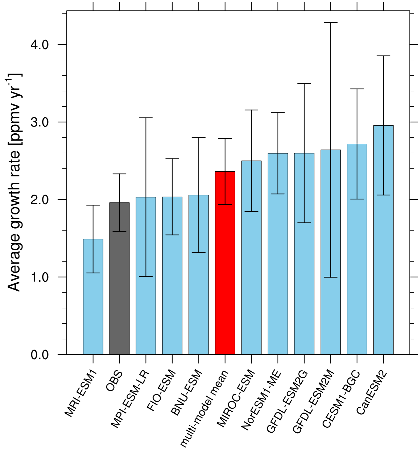
(b) CMIP5
