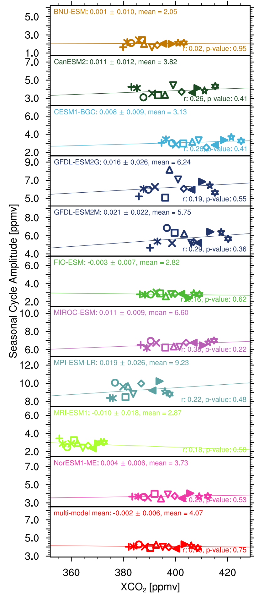
(a) SCIAMACHY mask
