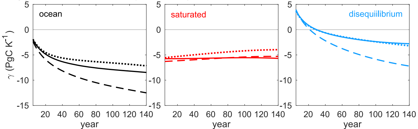
(d) carbon-climate feedback parameter, \gamma
