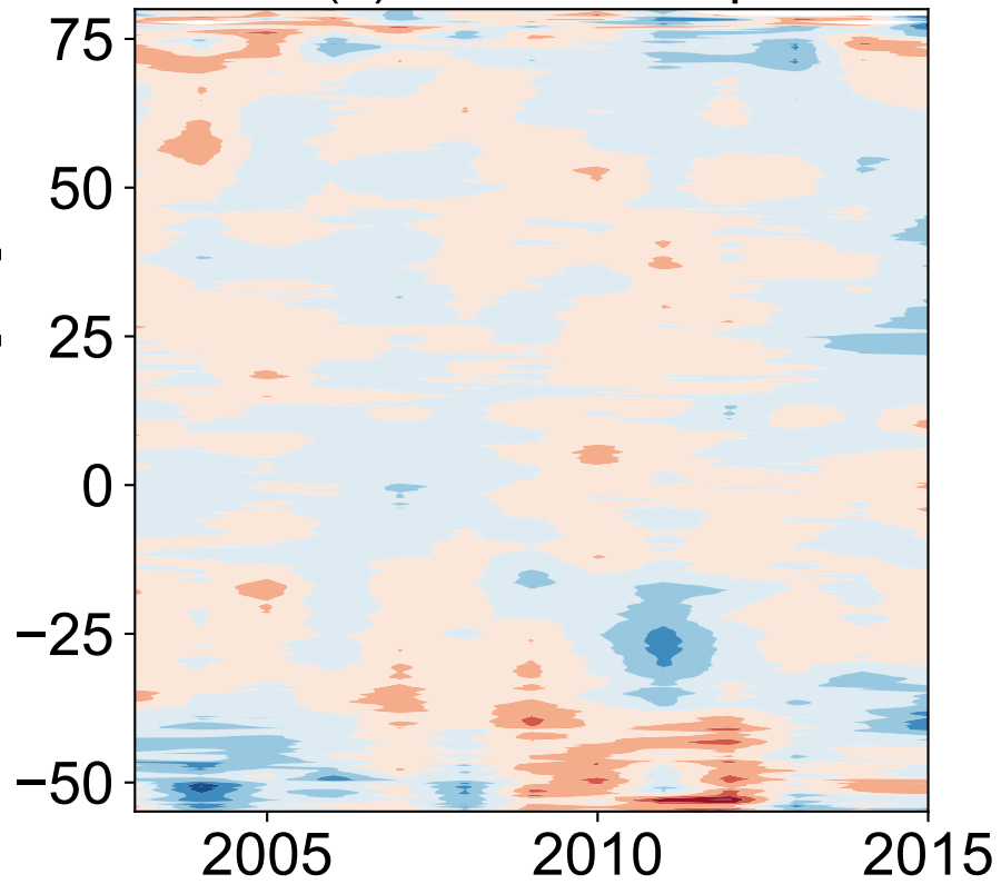
(a) GPPvodtemp
