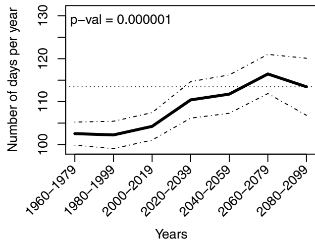
(d) PFT-MC under RCP 4.5
