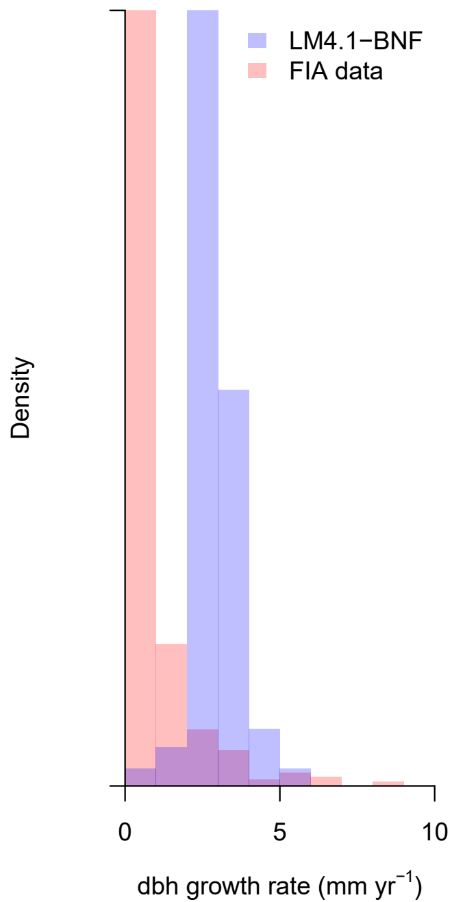
(b) Robinia
