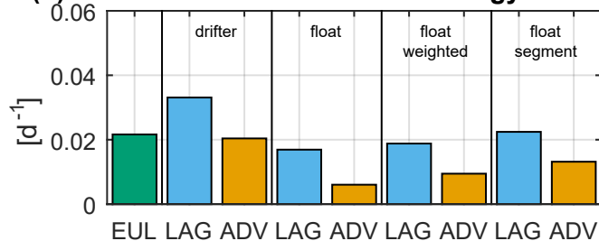
(d) metbio010d host bin -- climatology subtrahend
