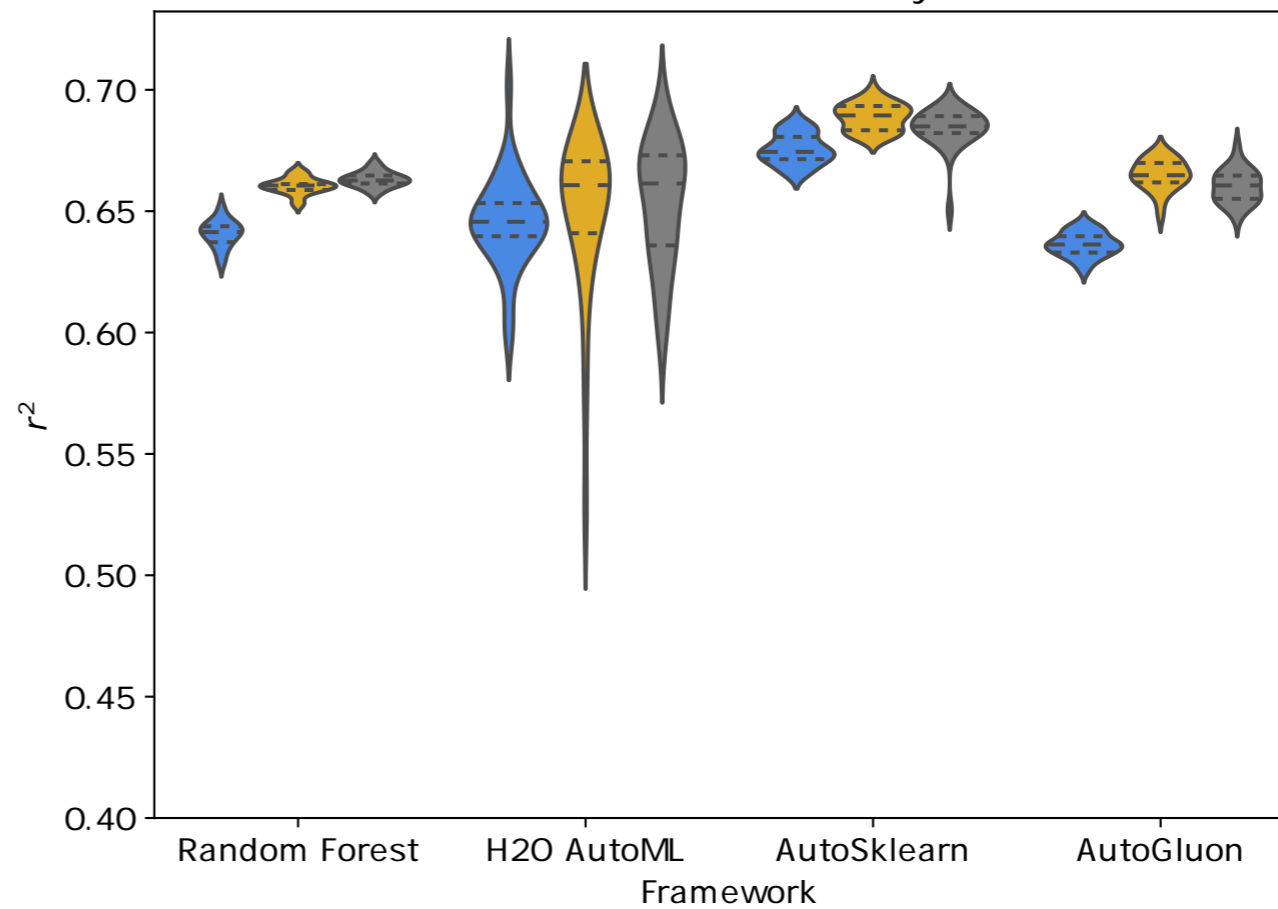
Anomalies
