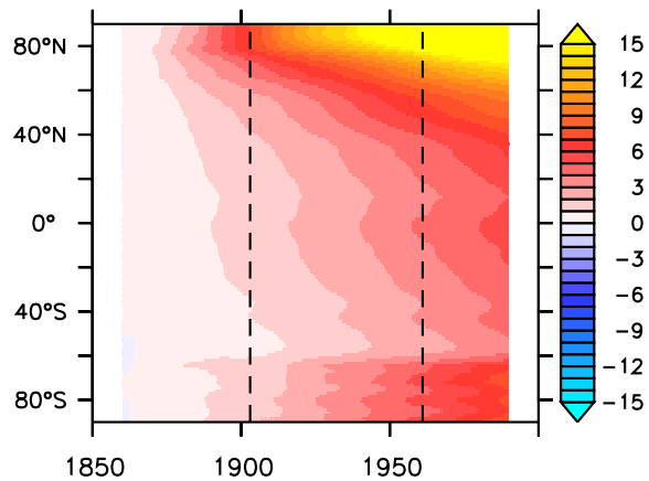
(g) UKESM 1pctCO2
