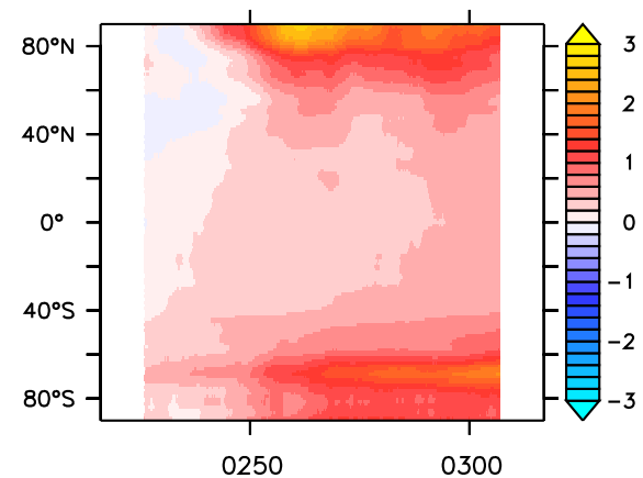
(f) MIROC ZEC2000
