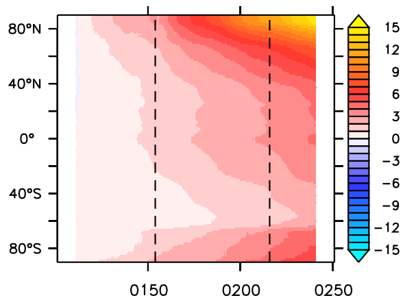
(d) MIROC 1pctCO2
