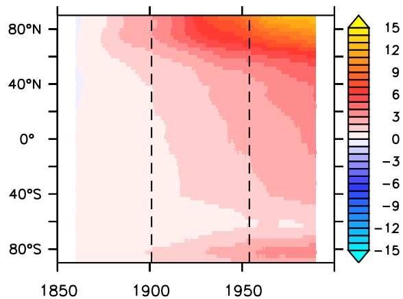
(d) MIROC 1pctCO2
