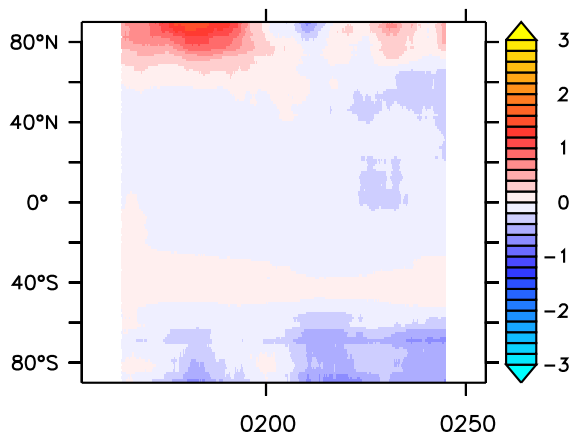
(e) MIROC ZEC750
