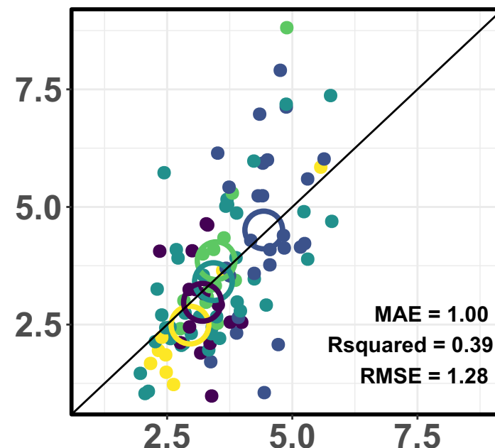
ER g C m -2 d -1
