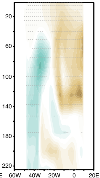
(d) NorESM2-MM
