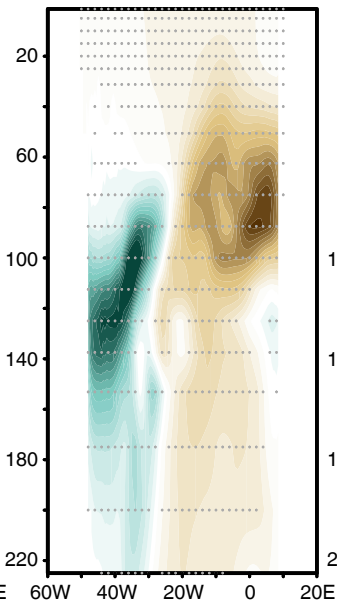
(b) NorESM1-AC
