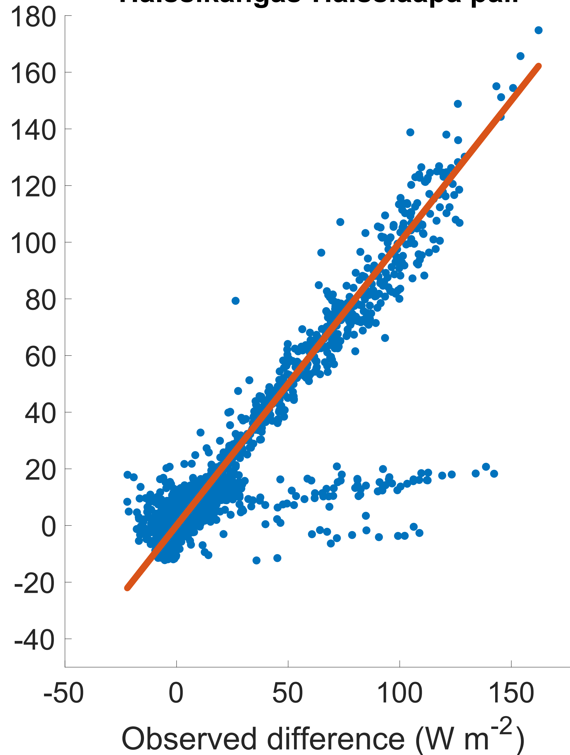
Halssikangas-Halssiaapa pair
