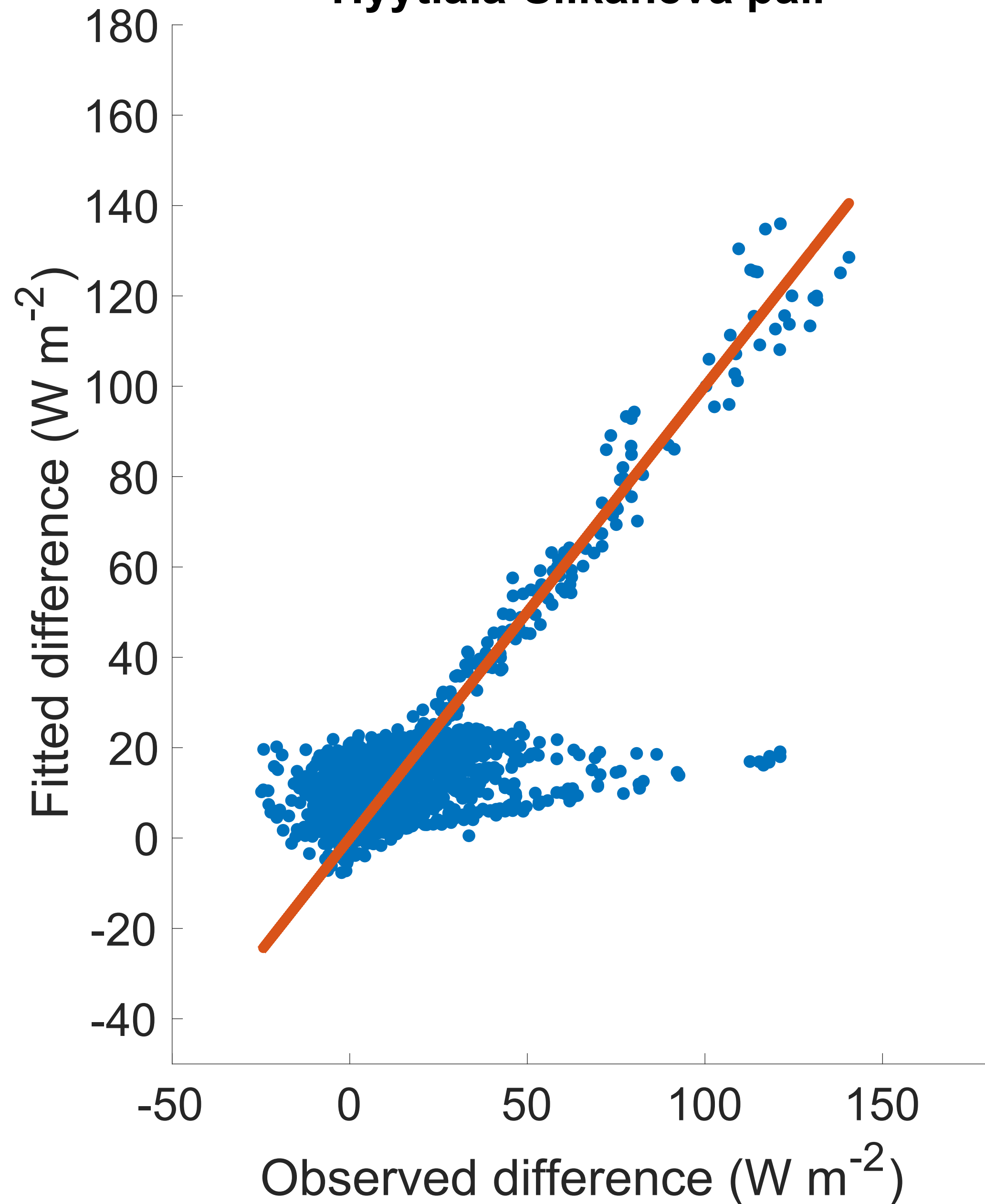
Hyytiälä-Siikaneva pair
