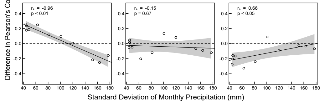
TROPOMI SIF
