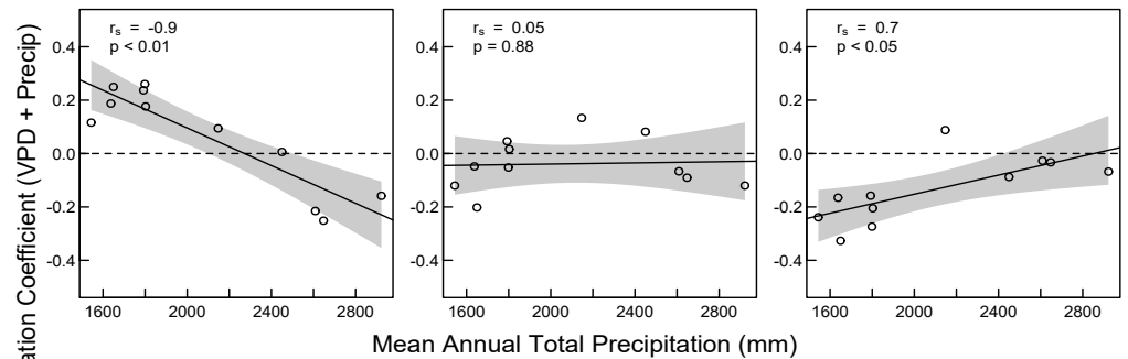
TROPOMI SIF
