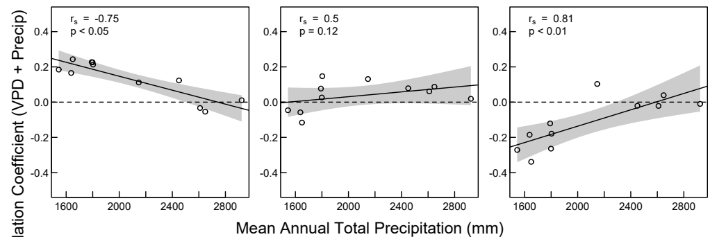
TROPOMI SIF
