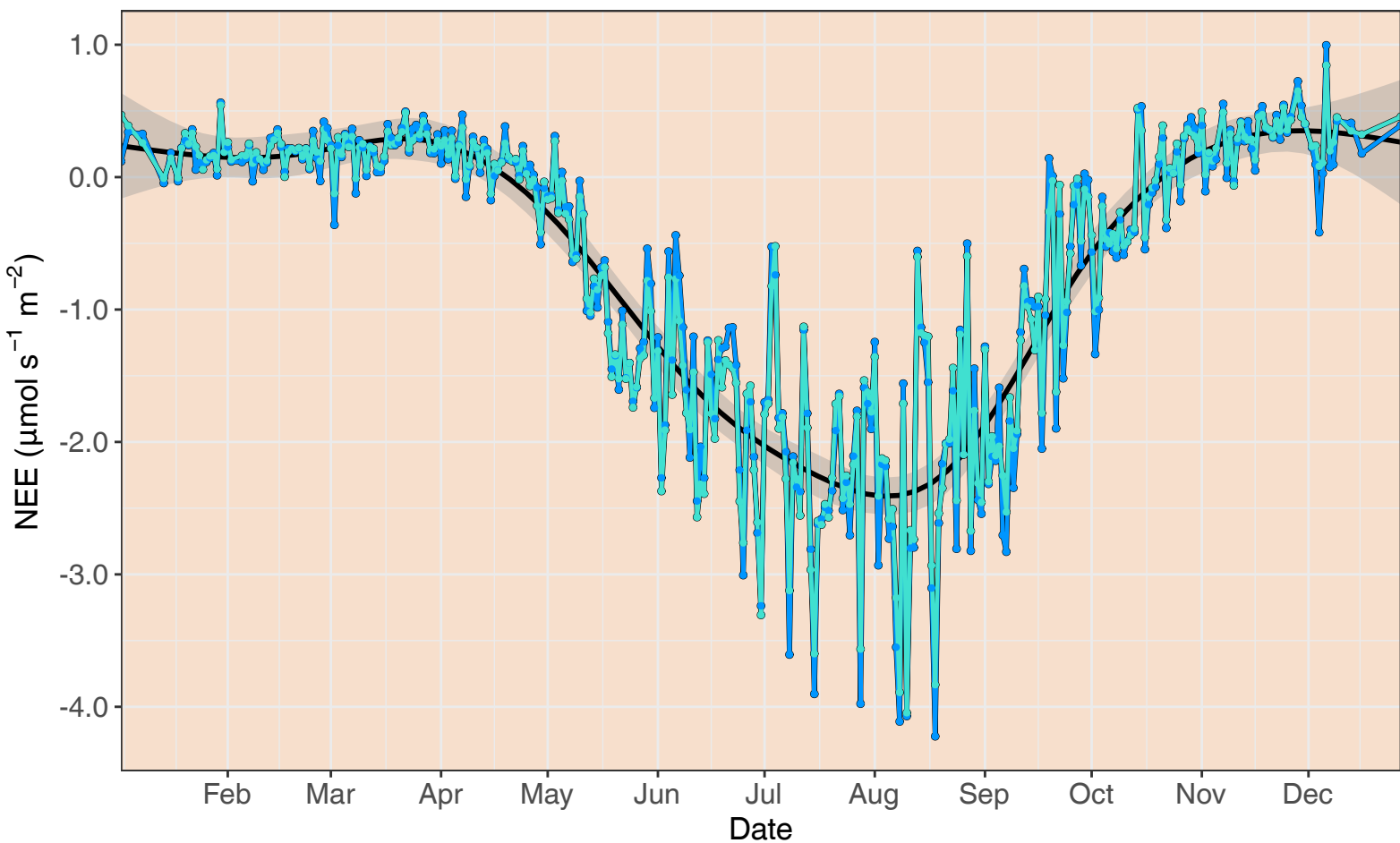
Värriö Daily Average, Actual and Modeled
