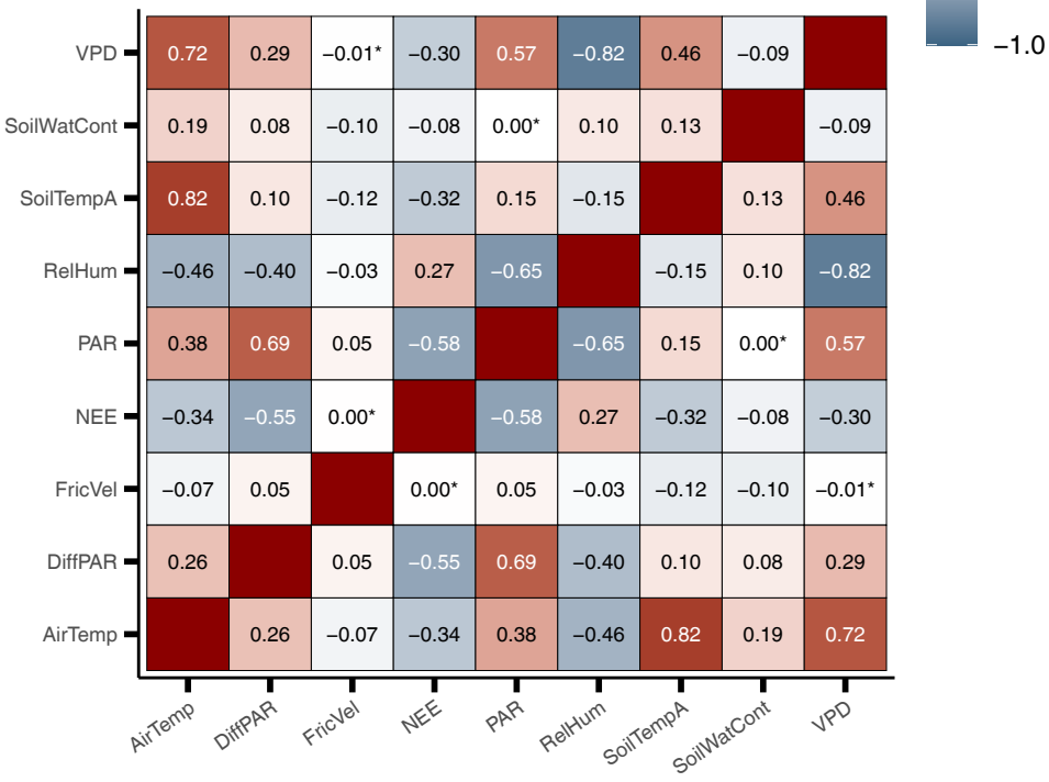
Correlation Matrix for Värriö
