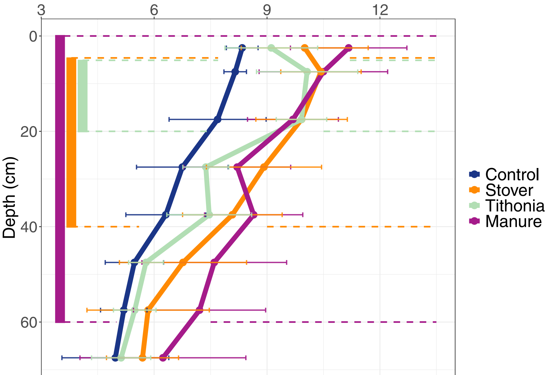
Carbon stocks per 5 cm layer (t ha -1 )
