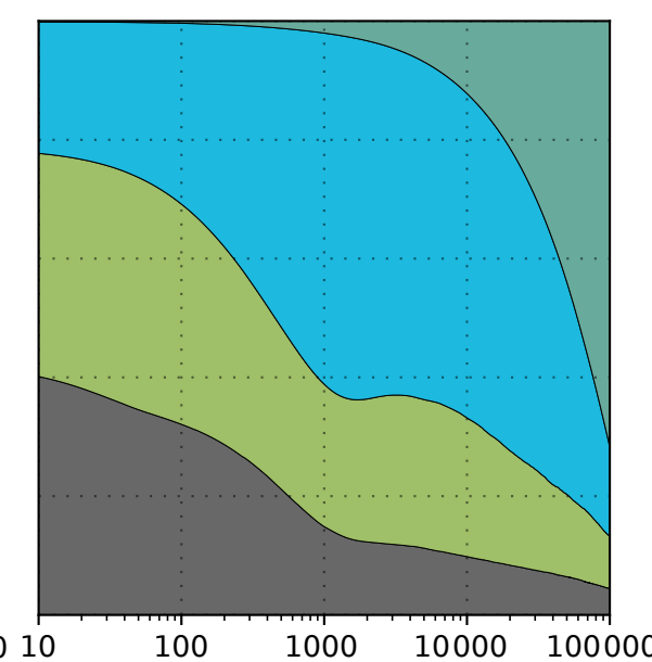
(b) 1000 PgC
