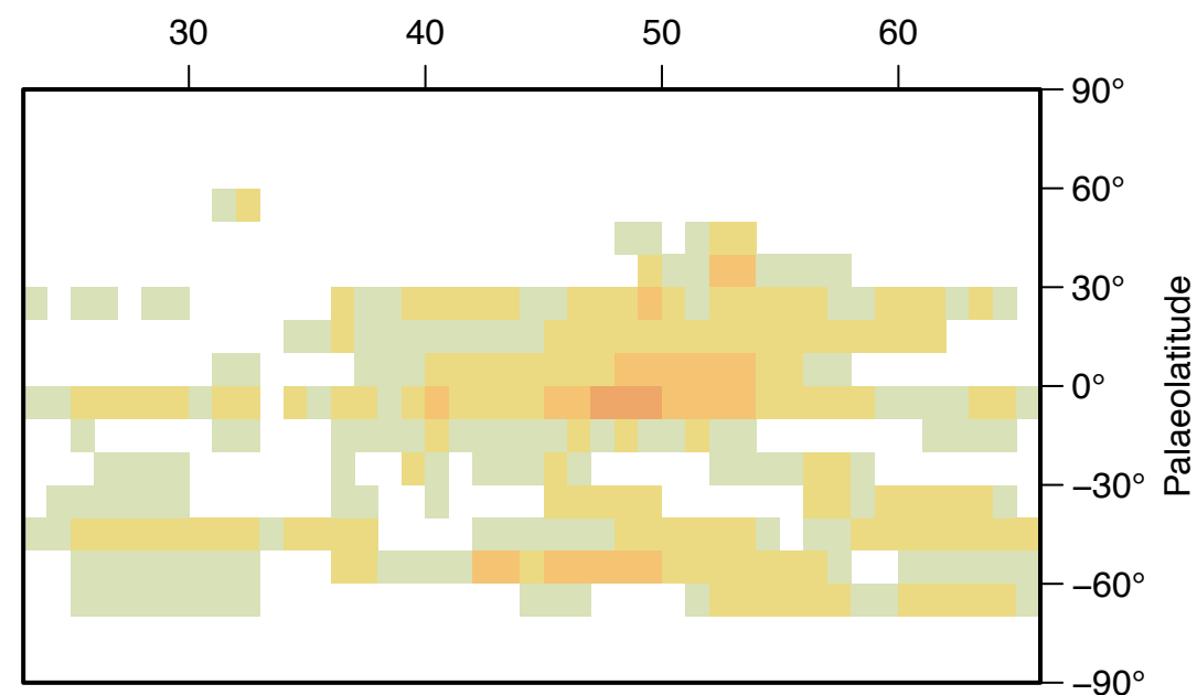
(d) Cherts (Muttoni & Kent, 2007)
