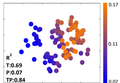
GCP-prog
