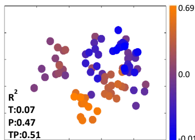
CLM45
