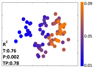
JULES
