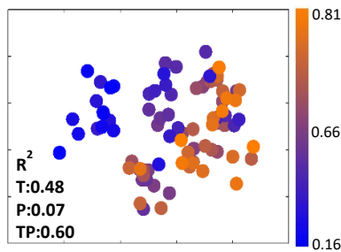
CLM5
