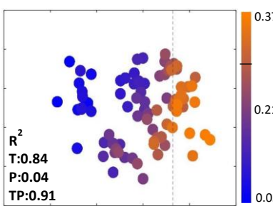
JSBACH-H
