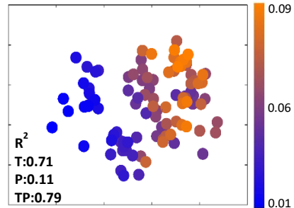
GCP-diag
