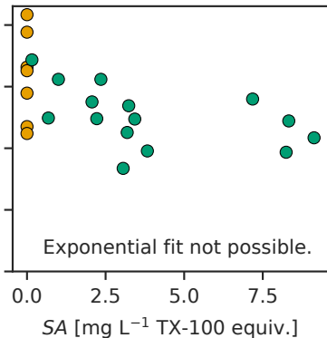
isoprene-d5
