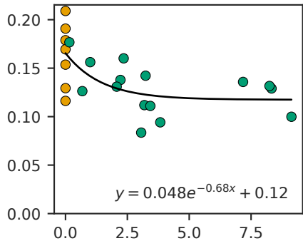
DMS-d3
