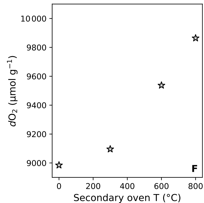
Lake Cadagno
