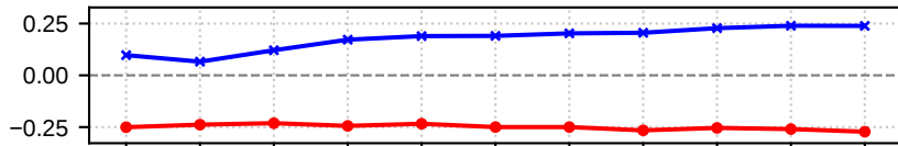
(d) SST (K)
