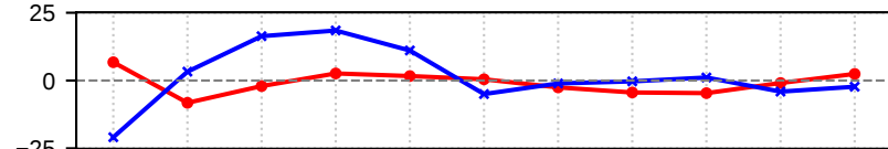
(e) SW ( \text{W m}^{-2} )
