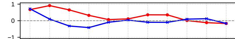
(g) WS ( \text{m s}^{-1} )
