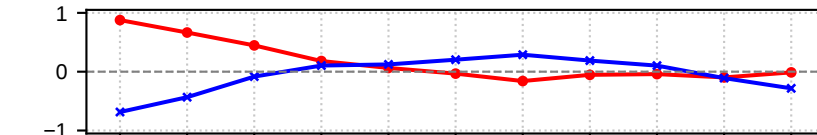
(o) WS ( \text{m s}^{-1} )
