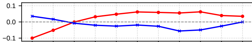
(a) Chl a ( \text{mg m}^{-3} )
