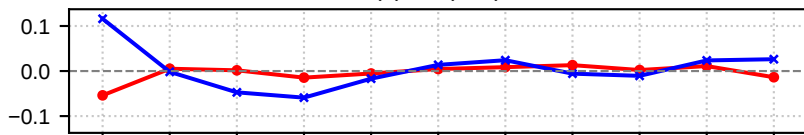
(h) TP (mm)
