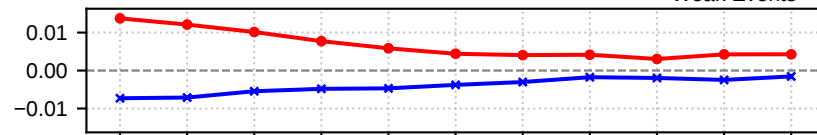
(i) Chl a ( \text{mg m}^{-3} )
