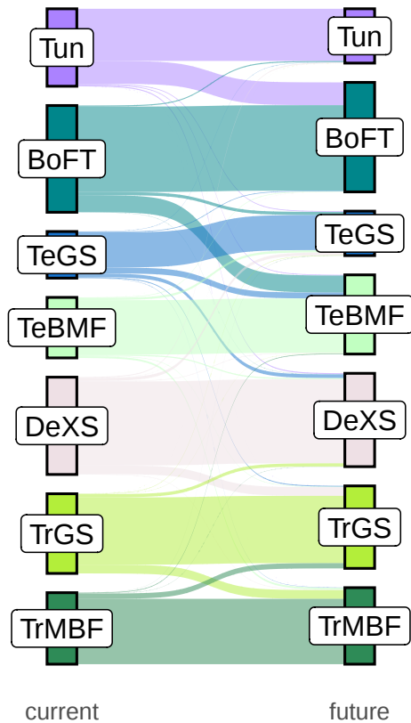
(b) RCP60
