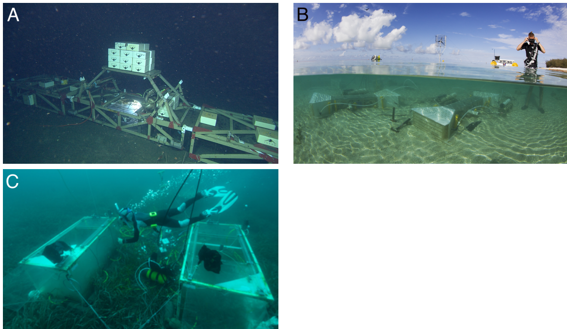
Fig. 4. A, deep-water FOCE (dpFOCE); B, Coral Proto FOCE (cpFOCE); C, European FOCE (eFOCE).
