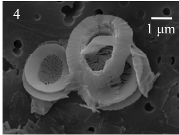
G. oceanica coccolith
