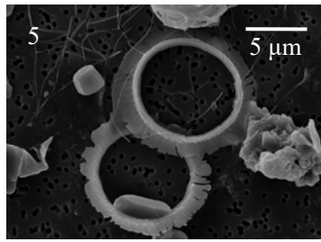
C. cristatus HET coccolithomorpha type
