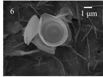
C. cristatus HET coccolithomorpha type
