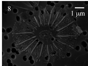
U. tenuis type I
